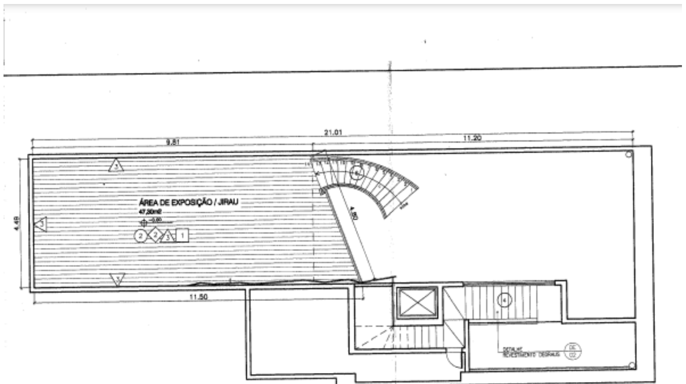
1 PLANTA BAIXA - JIRAU ESCALA 1:75
